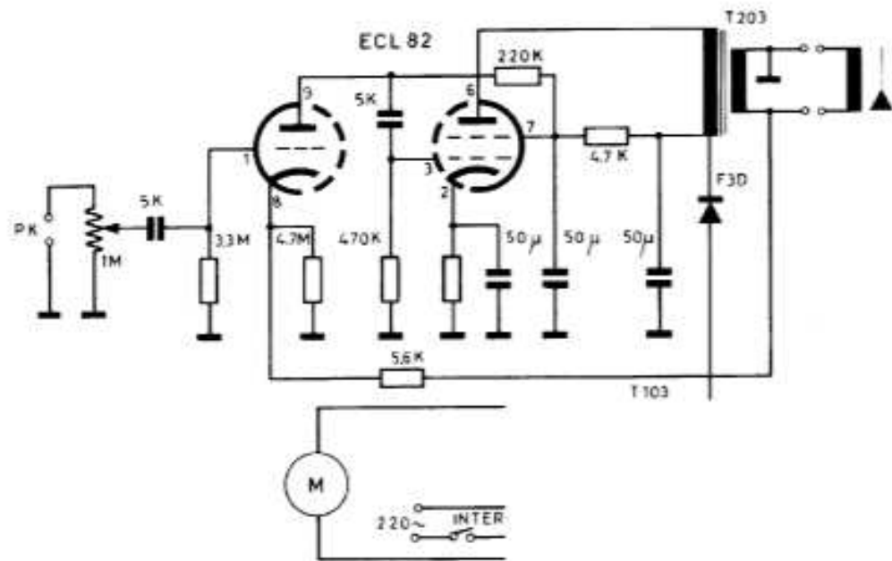
SCHEMA ELETTRICO DELLE FONOVOLIGIE FV/4 YORK e FV/6 CAMBRIDGE
